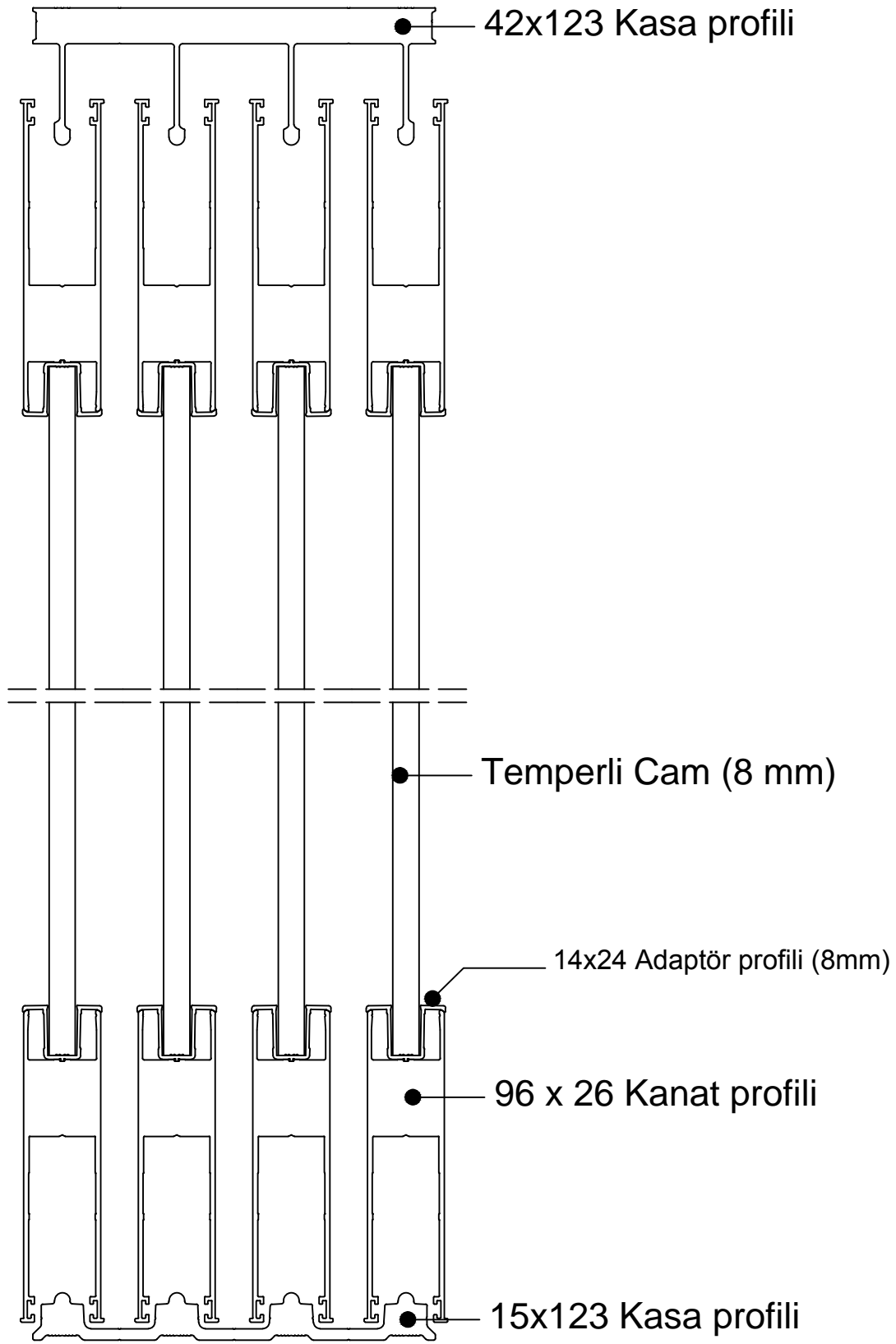
Slidemaster Flat 08 / Yan görünüş
